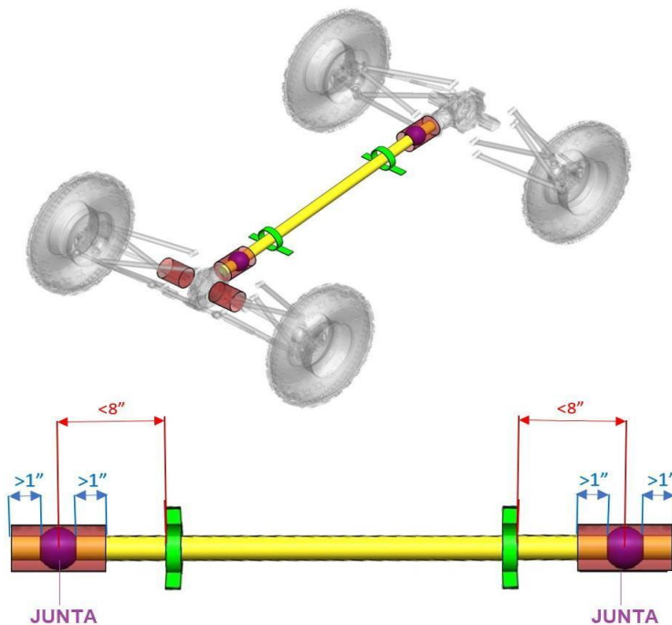
Figura 4 - Posição dos arcos de segurança de eixo cardan e dimensões anteparo de sistemas rotativos
