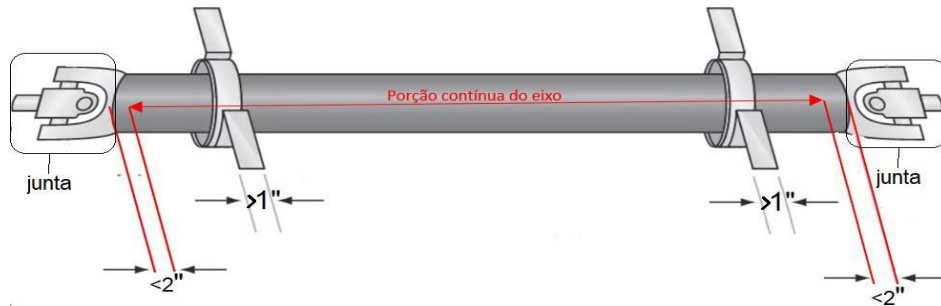
Figura 3 - Dimensões dos arcos de segurança de eixo cardan e porção contínua do eixo
