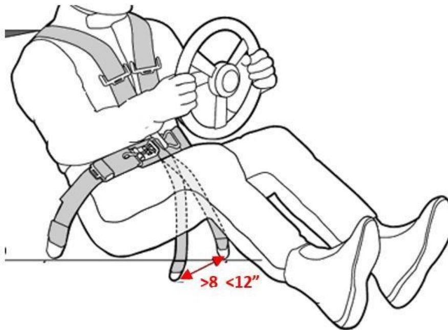
Figura 12 - Distanciamento das tiras anti submarinas para cinto de 6 pontos
