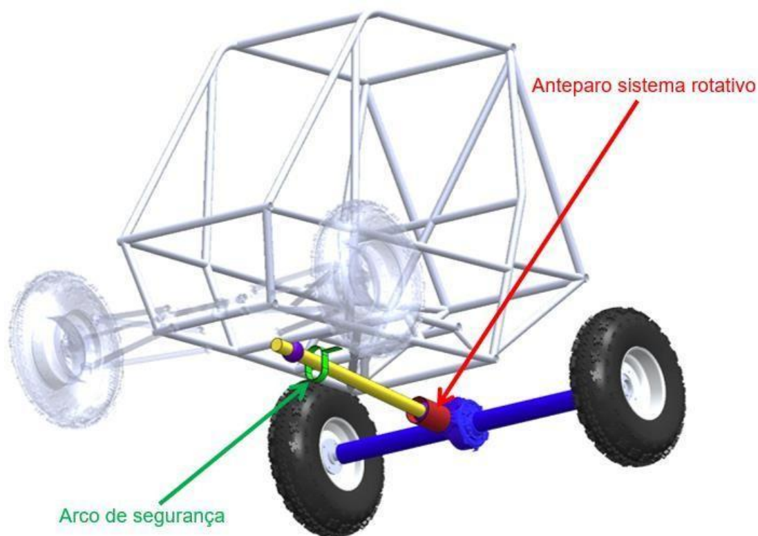
Figura 6 - Posição do arco de segurança de eixo cardan e anteparo para projetos com eixo de transmissão semi suspenso
