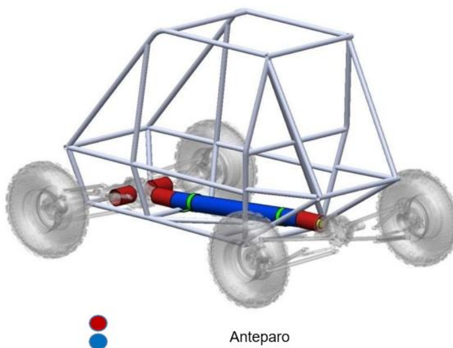
Figura 2 - Proteções dos sistemas rotativos no cockpit
