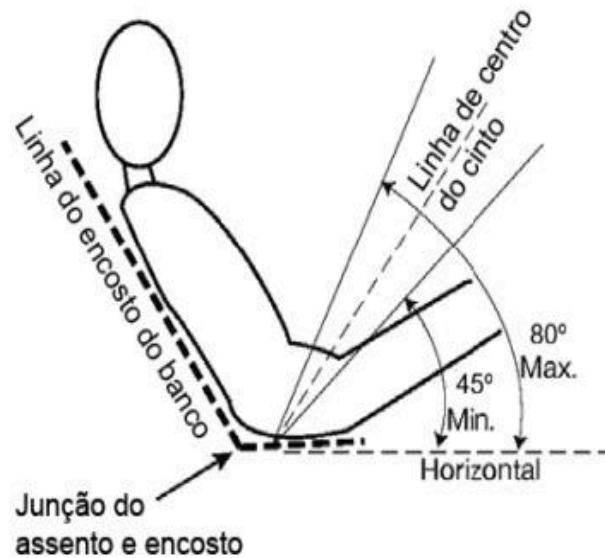
Figura B-44 – Posicionamento das tiras sobre a cintura
